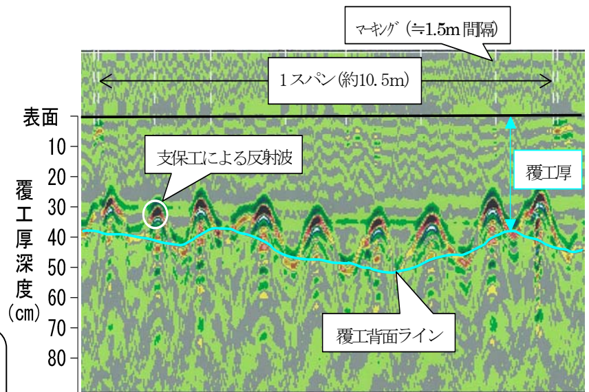
電磁波データトンネル覆工厚解析例
